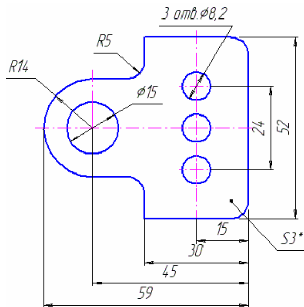
Рис. 3.10. Эскиз подвески
